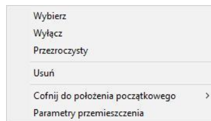
Chmury punktów
